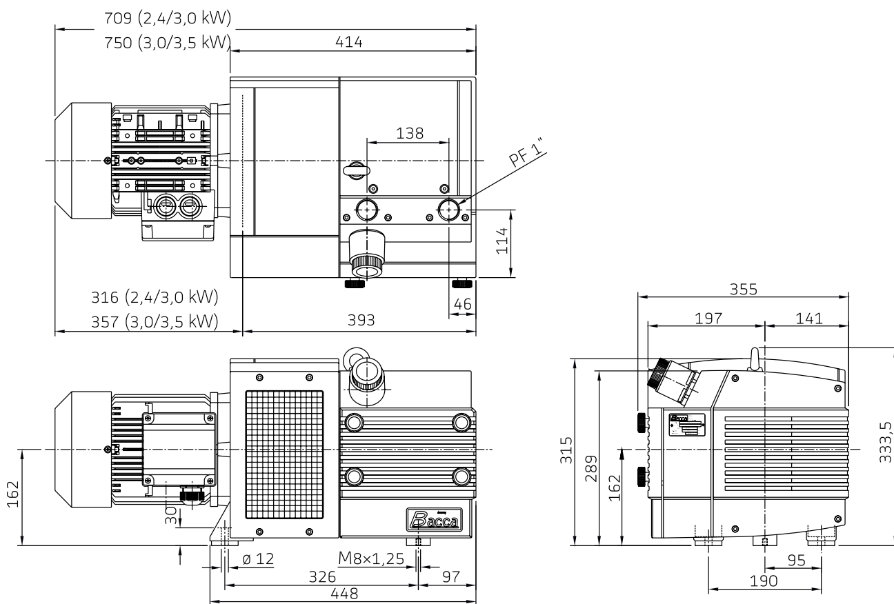
Lamelový rotační kompresor DRT 3140
